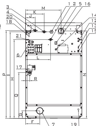
Задна страна
