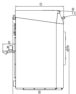
Лява страна
