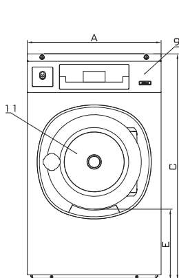
Предна страна
